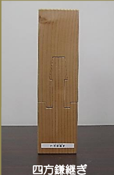
四方鎌継ぎ
